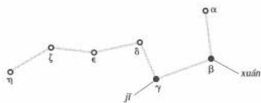
Xuánjī (21VC). Chariot (de la Grande Ourse). Les deux étoiles Xuán et Jī du chariot de la Grande Ourse.
