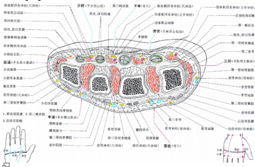
Coupe transversale passant par 8MC 8C 3IG 3TR et Willaogong - Yan Zhenguo 2002
